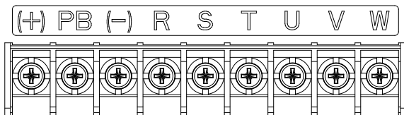
图 4-9 三相 380V 0022 (含) 以下主回路端子示意图
