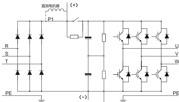
图 3-4 380V 0132 及以上主回路简图
