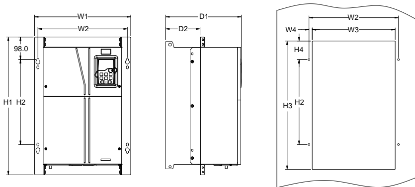
图 C-18 660V 22~132kW 法兰安装示意图
