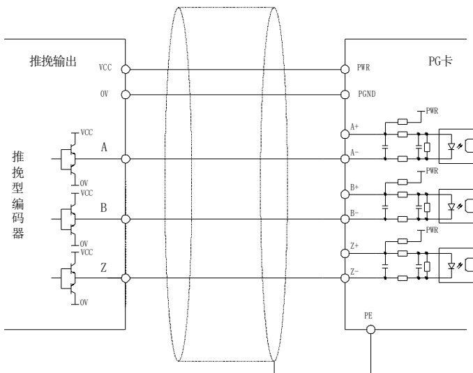
使用屏蔽线
