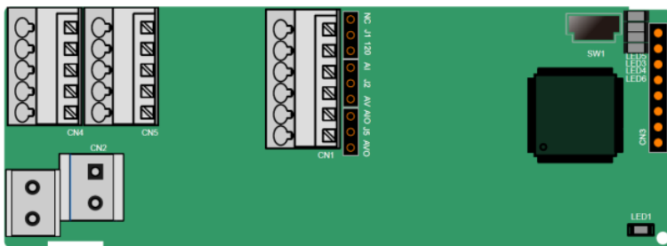
图 A-5 I/O 扩展卡 2 控制回路接线图
