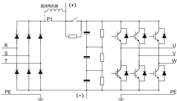
图 3-5 660V 主回路简图
