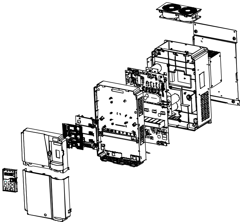
图 C-4 变频器结构图
