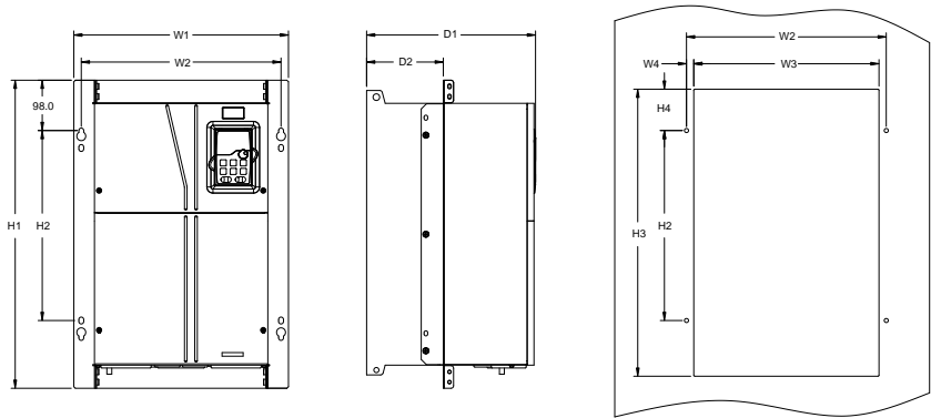
图 C-11 380V 0090~0110 法兰安装示意图
