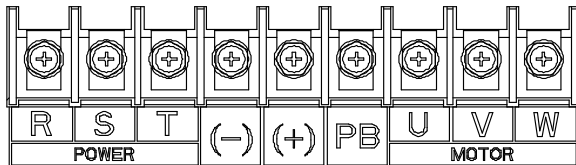
图 4-11 三相 380V 0045~0110 主回路端子示意图
