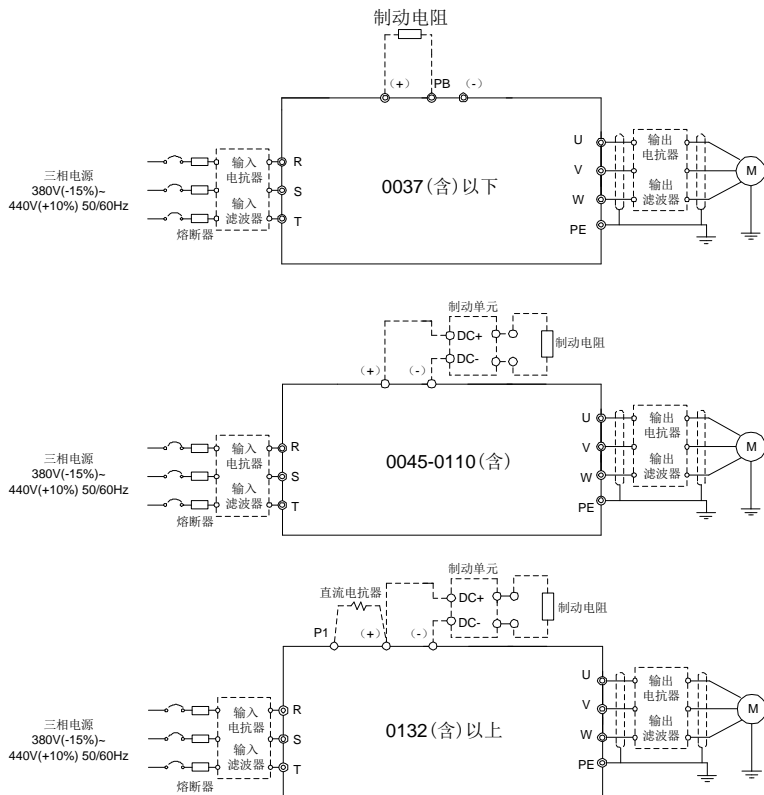
图 4-7 AC 3PH 380V(-15%)~440V(+10%)主回路接线图
