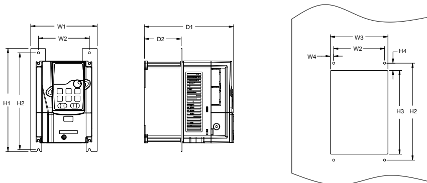
图 C-10 380V 01R5-0075 法兰安装示意图
