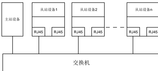
图 A-7 星型网络拓扑电气连接图
