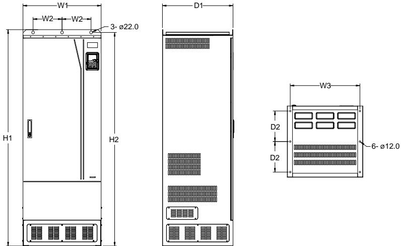
图 C-21 660V 400~630kW 落地安装示意图
