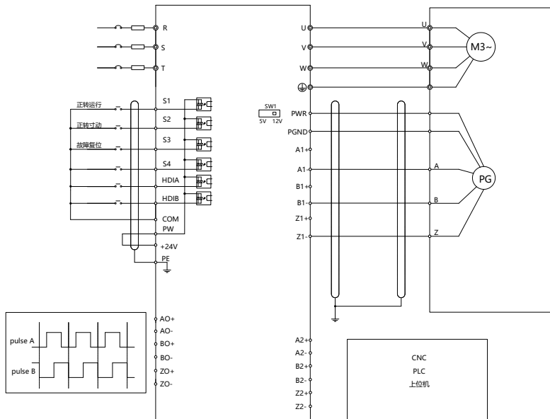
使用屏蔽线
