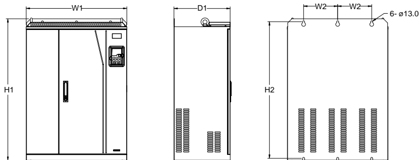
图 C-9 380V 0220-0315 壁挂安装示意图
