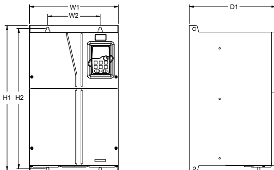
图 C-15 660V 22~132kW 壁挂安装示意图
