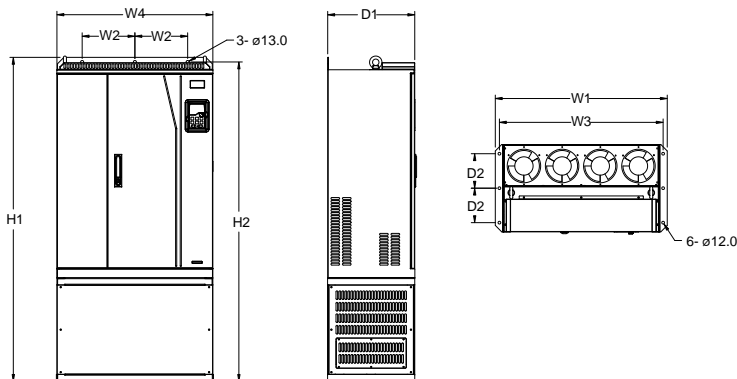
图 C-20 660V 250~355kW 落地安装示意图
