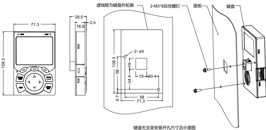
图 C-2 选配 LCD 键盘结构图
