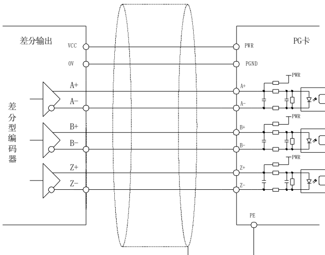
使用屏蔽线
