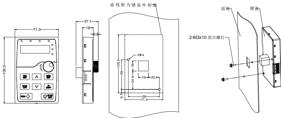
键盘无支架安装开孔尺寸及示意图
