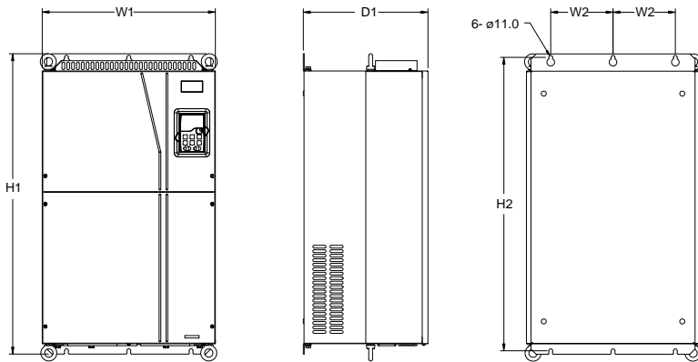
图 C-8 380V 0132-0200 壁挂安装示意图
