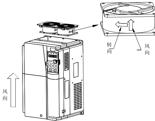
图 9-1 7.5kW (含) 以上机器风扇维护示意图
