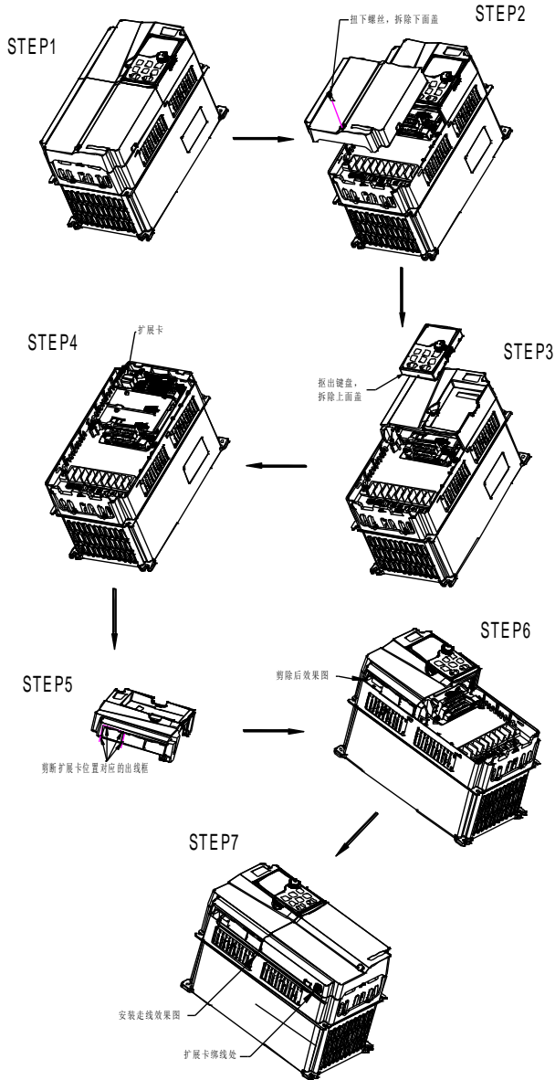
图 A-3 扩展卡接线安装步骤示意图
