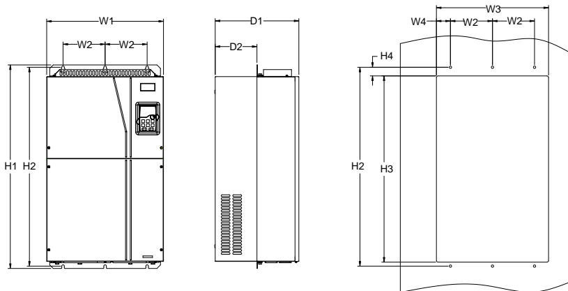
图 C-19 660V 160~220kW 法兰安装示意图
