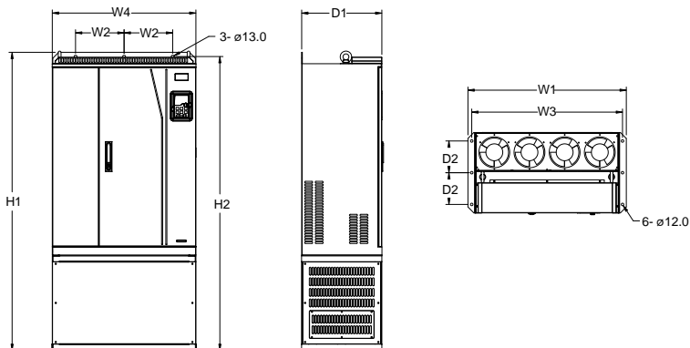
图 C-13 380V 0220~0315 落地安装示意图
