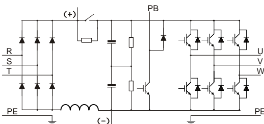
图 3-2 380V 0018~0037 主回路简图
