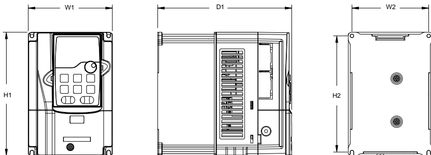
图 C-5 380V 01R5-0037 壁挂安装示意图
