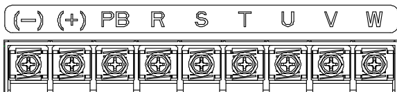
图 4-10 三相 380V 0030~0037 主回路端子示意图
