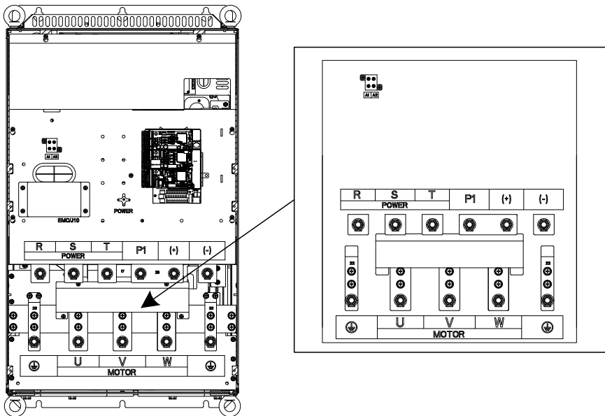
图 4-14 380V 0132-0200、660V 160-220kW 主回路端子示意图
