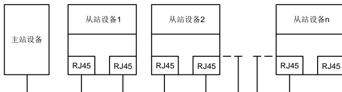
图 A-6 线型网络拓扑电气连接图
