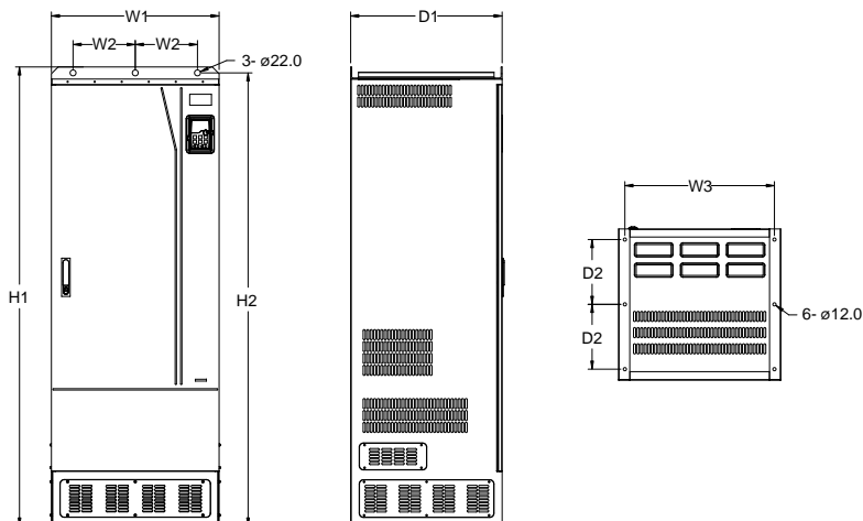
图 C-14 380V 0355~0500 落地安装示意图
