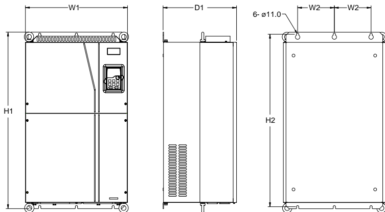
图 C-16 660V 160~220kW 壁挂安装示意图
