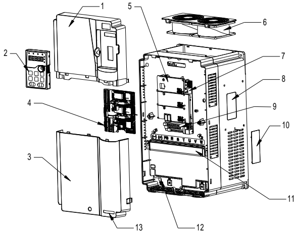
图 3-8 产品结构示意图
