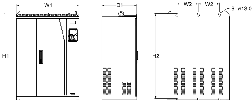
图 C-17 660V 250~355kW 壁挂安装示意图
