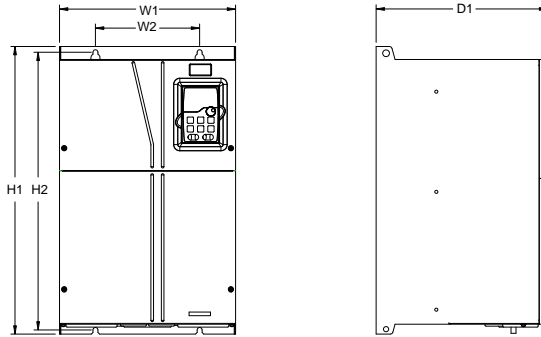
图 C-7 380V 0090-0110 壁挂安装示意图
