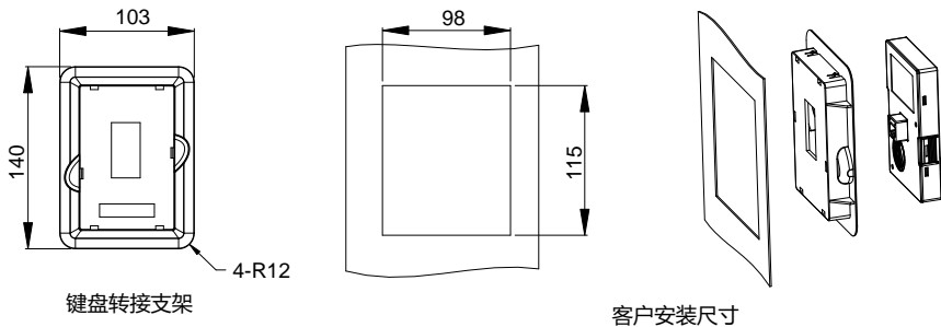
图 C-3 380V 01R5-0500、660V 22-630kW 键盘安装架（选配）图
