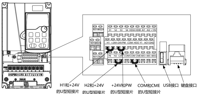
图 4-19 U 型短接位置示意图
