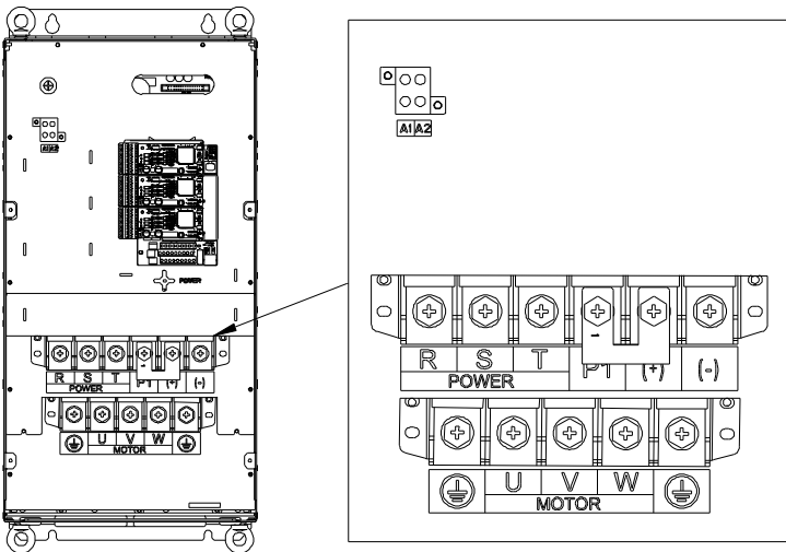
图 4-13 660V 55~132kW 主回路端子示意图
