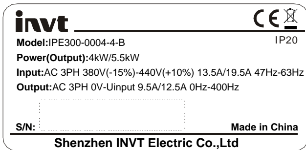
图 3-6 产品铭牌
