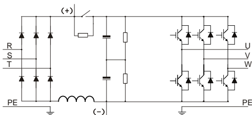
图 3-3 380V 0045~0110 主回路简图
