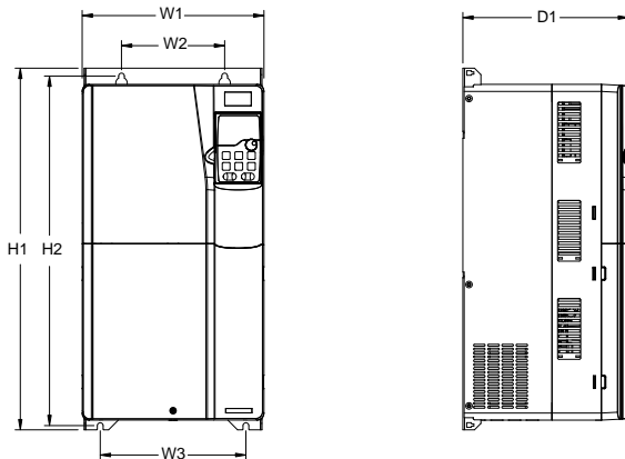
图 C-6 380V 0045-0075 壁挂安装示意图
