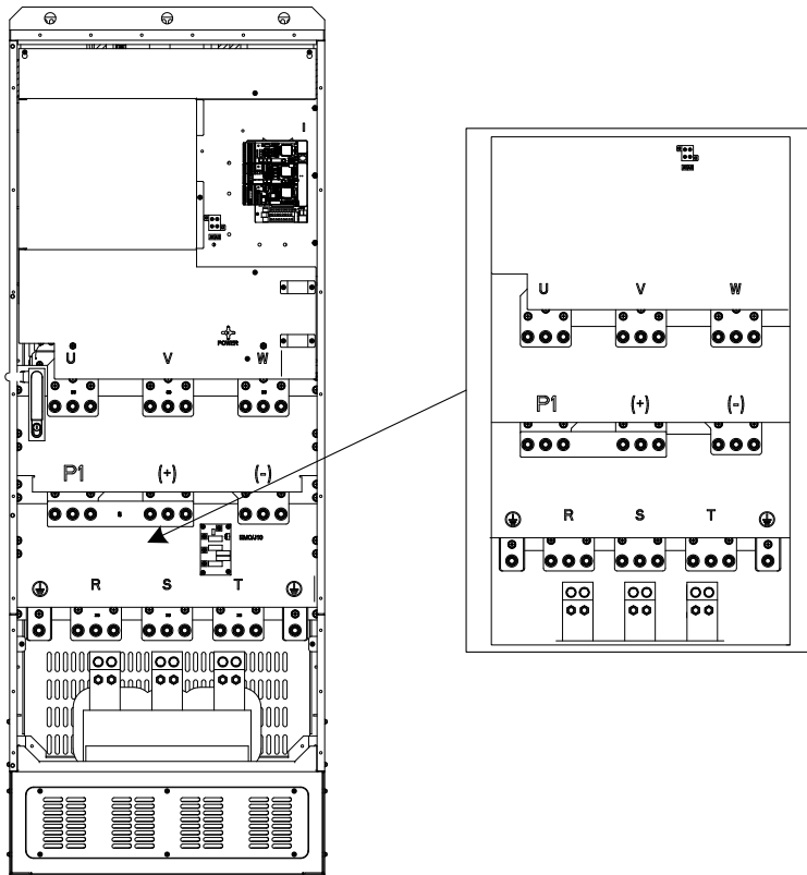
图 4-16 380V 0355~0500、660V 400~630kW 主回路端子示意图
