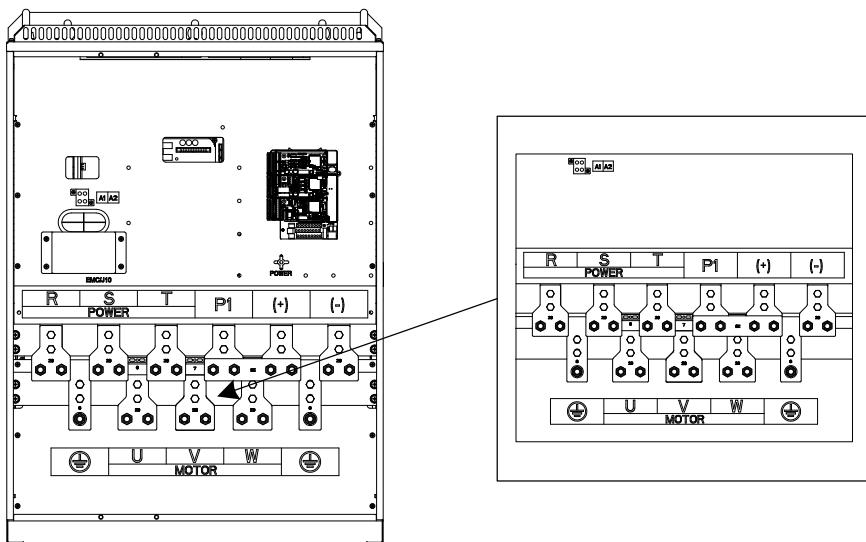
图 4-15 380V 0220-0315、660V 250-355kW 主回路端子示意图
