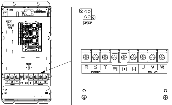
图 4-12 660V 22~45kW 主回路端子示意图
