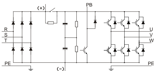
图 3-1 380V 0015 及以下主回路简图
